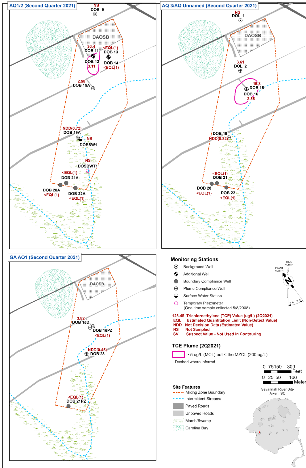
Figure B-7. DOSB TCE Concentrations in AQ1/2, 3 and GA AQ1, 2021
