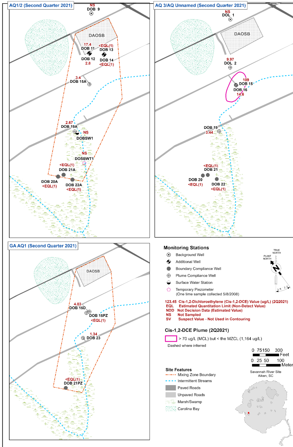
Figure B-8. DOSB cis-1,2-DCE Concentrations in AQ1/2, 3 and GA AQ1, 2021
