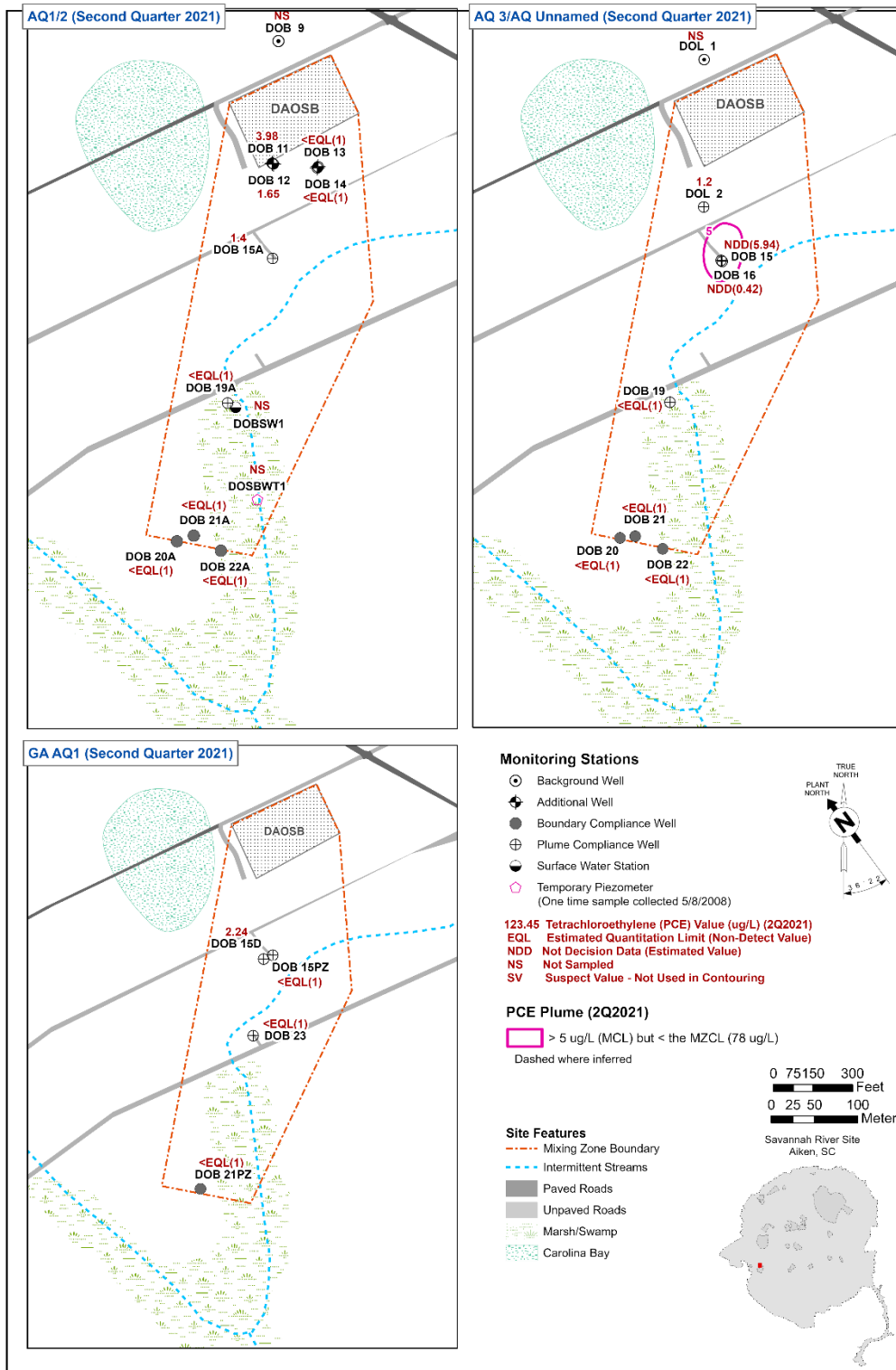
Figure B-6. DOSB PCE Concentrations in AQ1/2, 3 and GA AQ1, 2021
